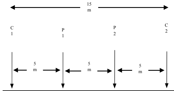
Gambar 1. Skema Penelitian Konfigurasi Wenner (Armanto Zet T. S, 2020)
